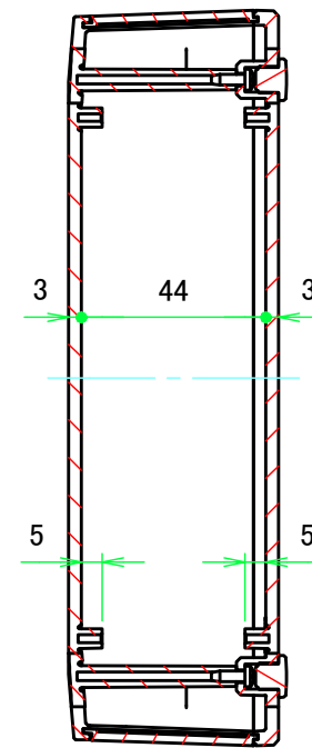
A-A (1:2)
