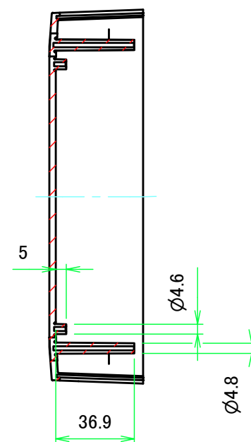
C-C ( 1 : 2.5 )
