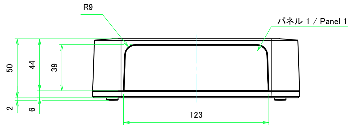
B-B (1:2)
