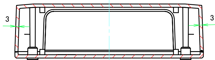
B-B (1:2)
